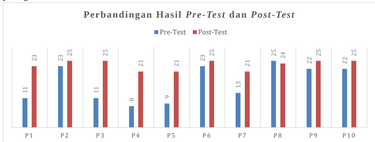
Gambar 3 Perbandingan Hasil Pre-Test dan Post Test
