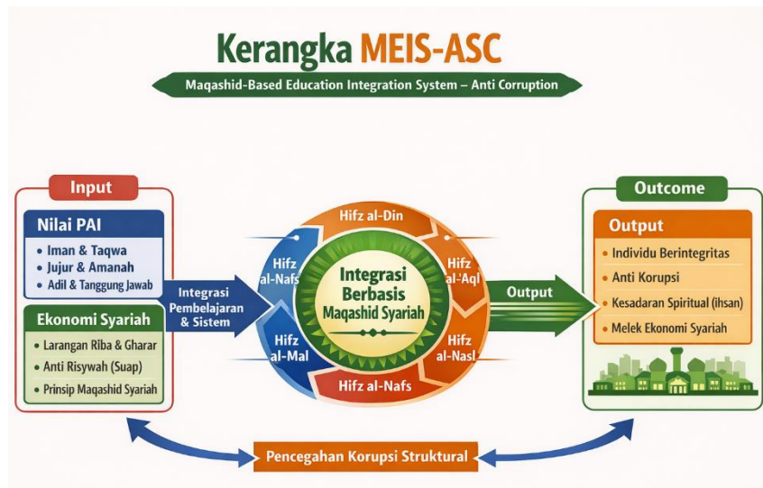
Gambar 5. Kerangka MEIS-ASC
