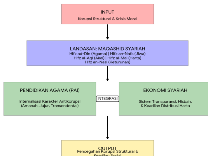
Gambar 2. Kerangka Berfikir
